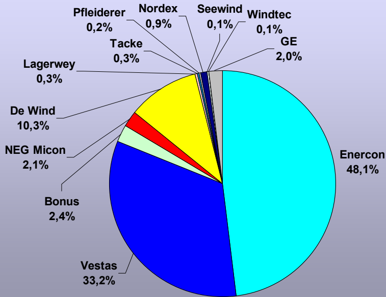
Marktanteile Österreich gesamt installierte Windkraftleistung 1994 - 2004 (606 MW)
