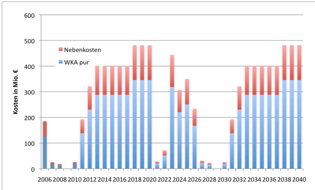
Abbildung 40: Investitionskosten für Windkraftanlagen
