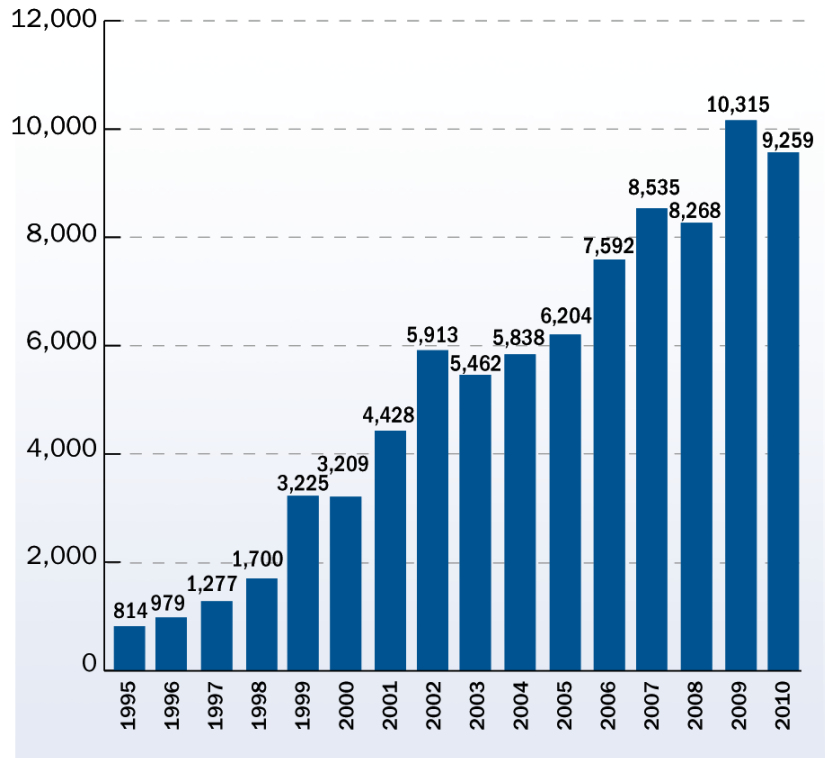
Abbildung 14: Jährlich installierte Windkraft in der EU (Quelle: EWEA 2010b)
